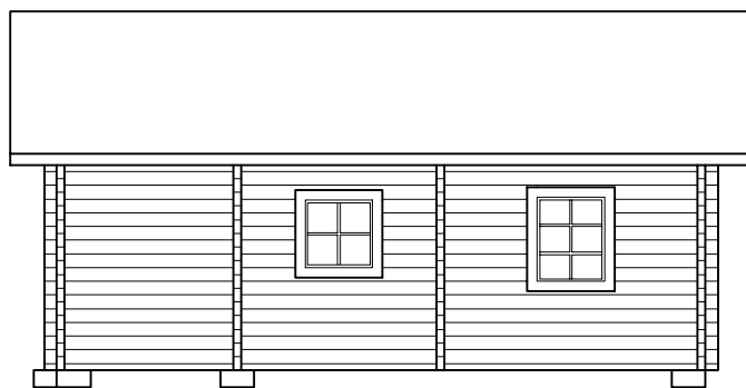
Höger
