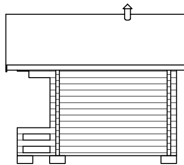
Höger
