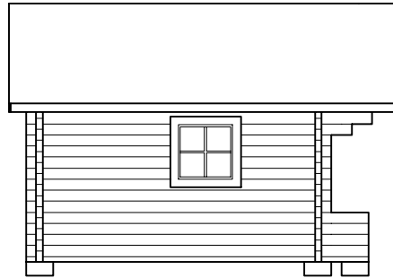
Vänster
