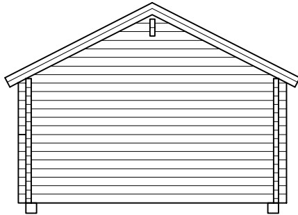
Baksida
